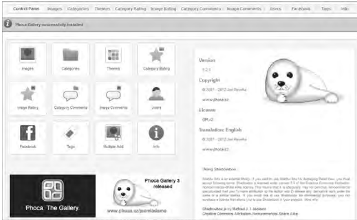
FIGURE 14.2 : Tableau de bord de Phoca Gallery, en anglais.
