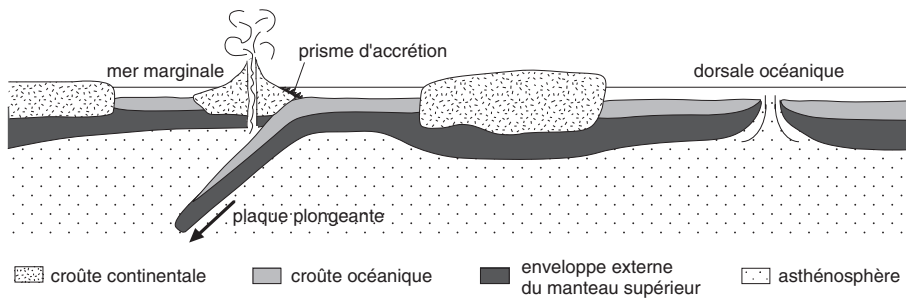
Figure 1.2 – Schéma synthétique simplifié du mécanisme de la tectonique des plaques.
